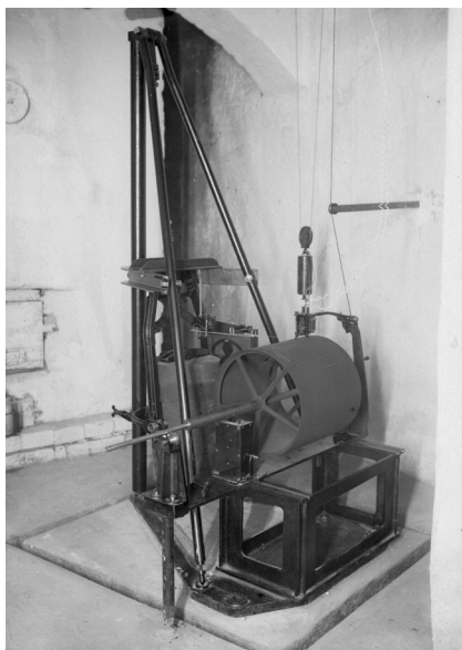
A kolozsvári egyetemi földrajzi intézet Mainka-féle földrengésjegyzőkészüléke (1912) [Kol1066] N-S komponens [Kol1067] E-W komponens
